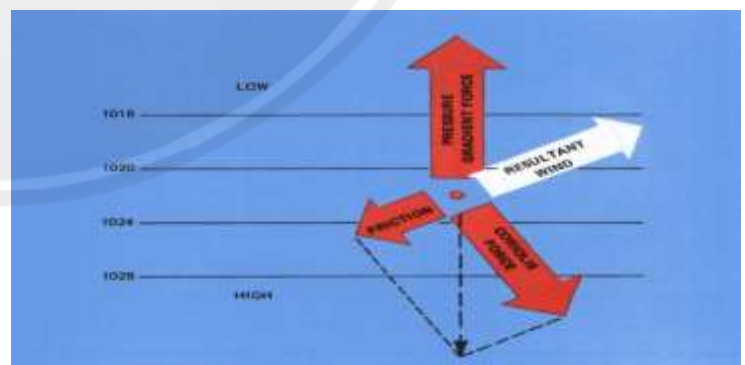
Coriolis Force
